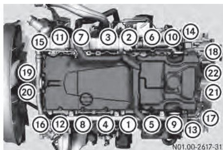
6R 1000 の締め付け順序
