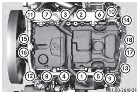
4R 1000 の締め付け順序
